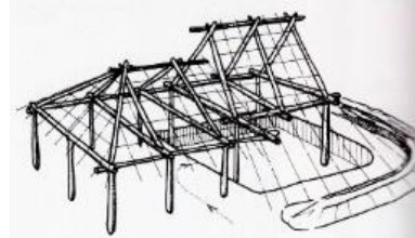
掘立柱付竪穴住居復元図
